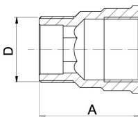
FT216 Prodloužení kované Forged flanged connection
